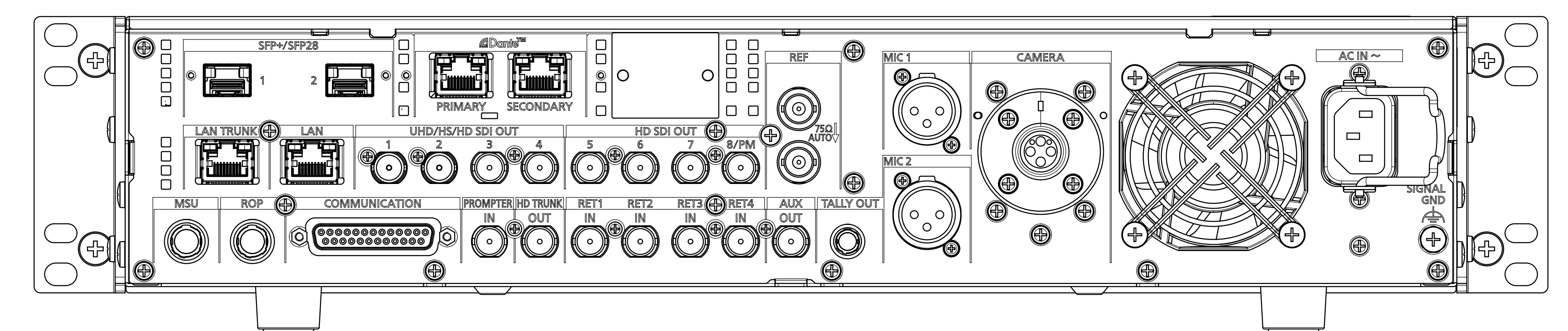
REAR_VIEW
