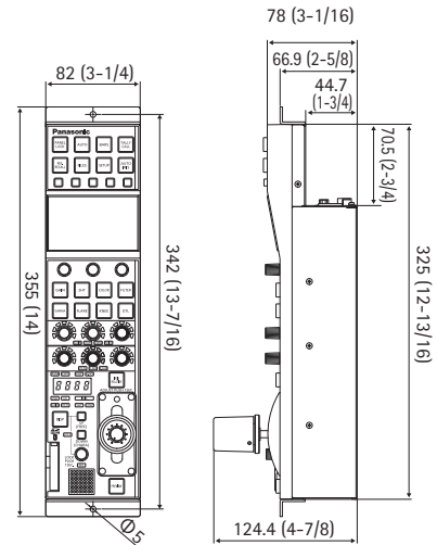
■ AK-HRP1005GJ
