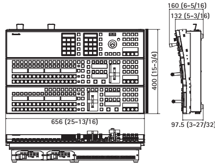
Mainframe
