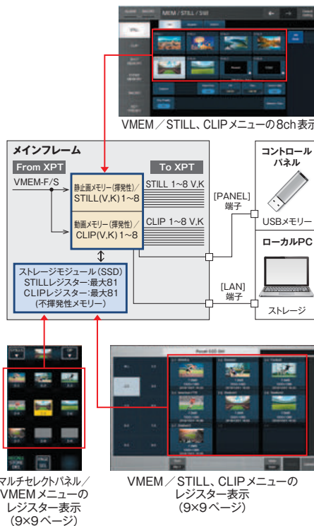
ビデオメモリーの構成とメニュー表示（AV-HS8300）
