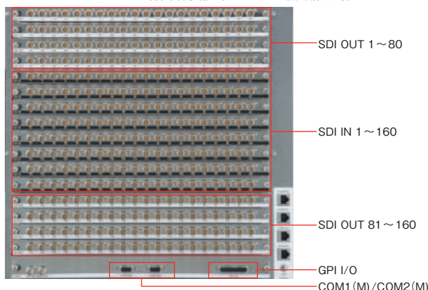
AV-WM8400 Series 背面端子部 (オプション最大構成時)
