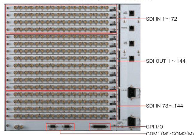
AV-WM7400 Series 背面端子部 (オプション最大構成時)
