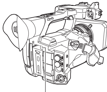
Akku-Entriegelungstaste
