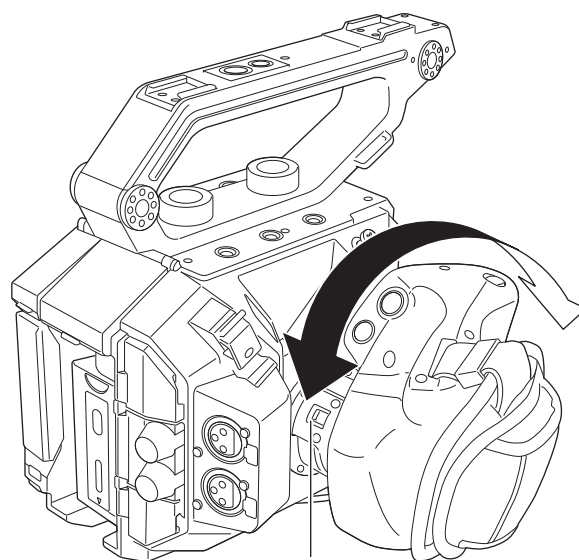
Levier de rotation de la poignée
