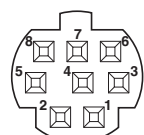
Connecteur RS-232C IN/OUT
